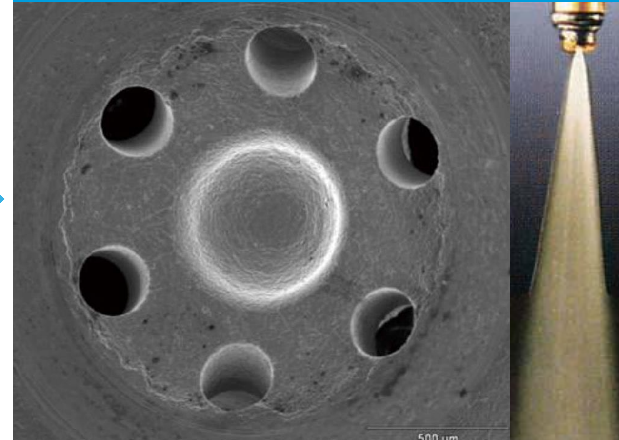
洗浄された燃料噴射口と回復した燃料噴射パターン
