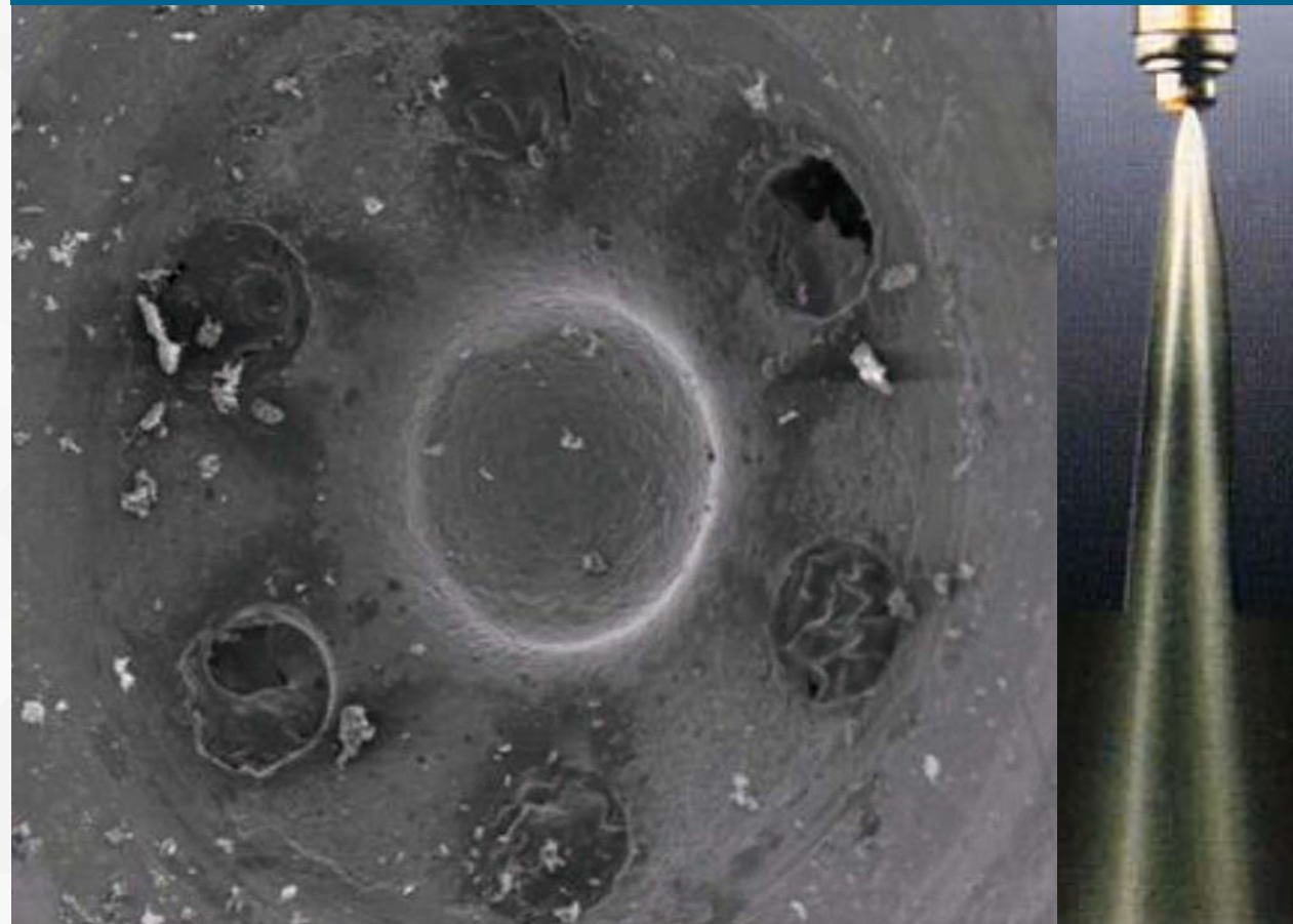
堆積物により詰まりが見える燃料噴射口と乱れた燃料噴射パターン
